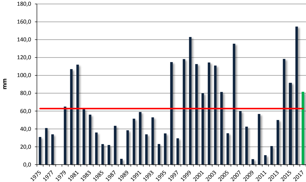
Gráfico 1: Promedio histórico 62.8 mm (línea roja).
