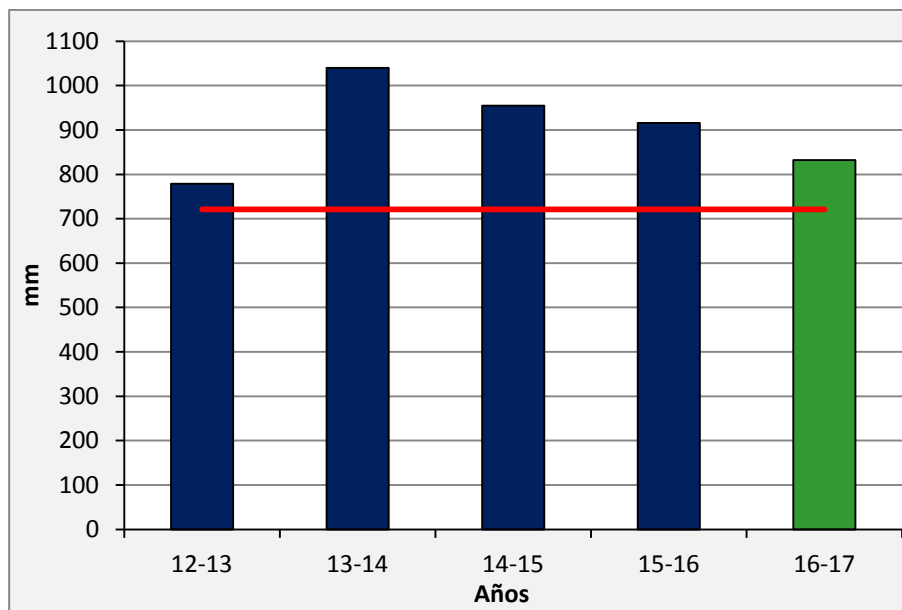
Gráfico 2: Acumulación de precipitaciones durante el periodo julio-abril (línea roja: 721.2 mm, promedio histórico).
