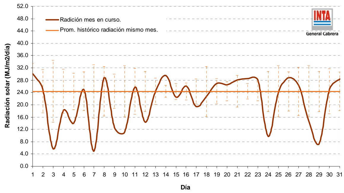
Gráfico 5: Evolución de la radiación solar del mes en curso ( serie curvilíneas ) y radiación media histórica del mismo mes ( serie rectas ) para el periodo 2001-2015. Las líneas sobre la recta histórica, representan el desvío estándar diario de la serie.
